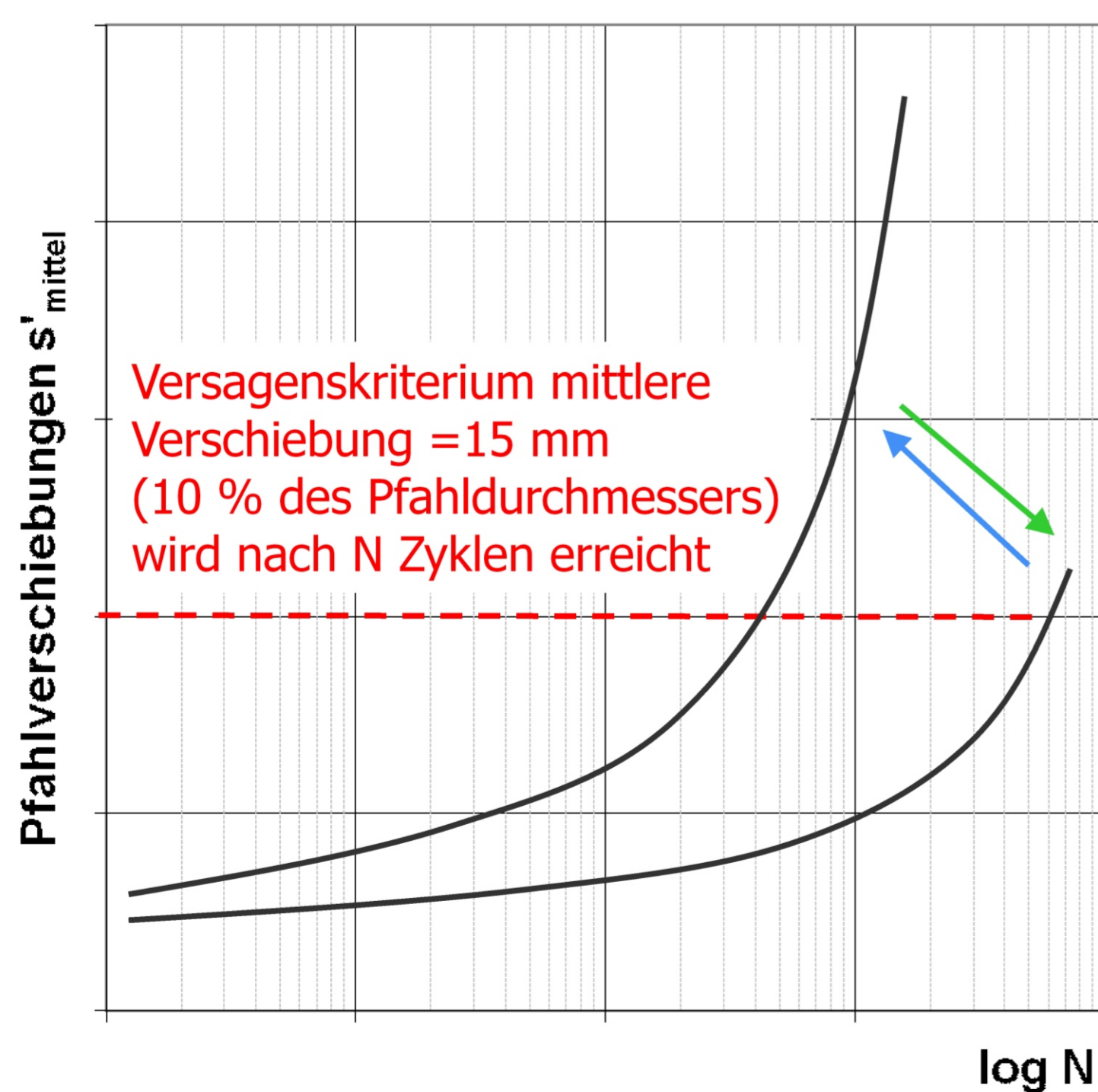
Pfahlverschiebungen für Zugschwell- und Wechselastversuche Pile displacements (one-way and two-way cyclic loading)
