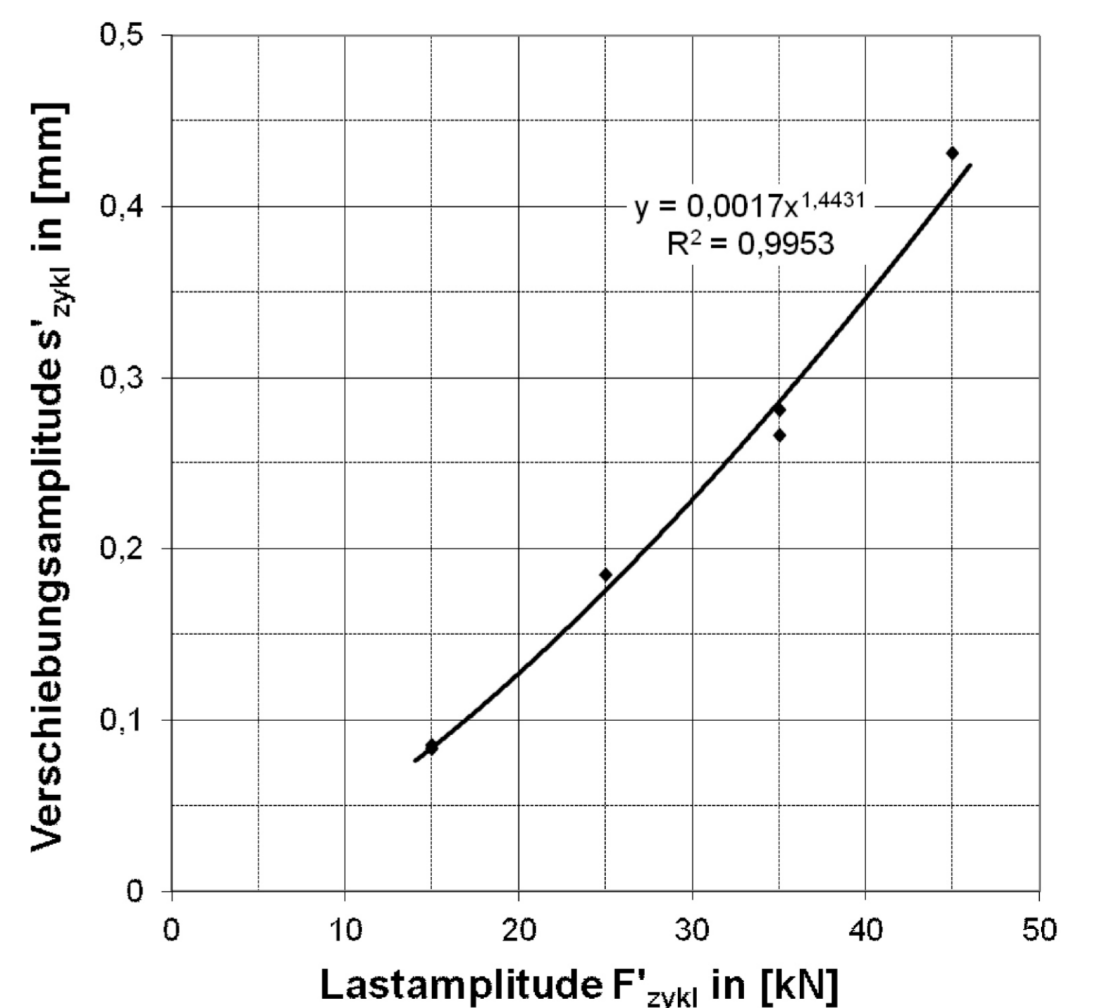
Abhängigkeit der Verschiebungsamplitude von der Lastamplitude bei Zugschwellastversuchen Displacement amplitude vs. load amplitude for one-way cyclic loading (tension)
