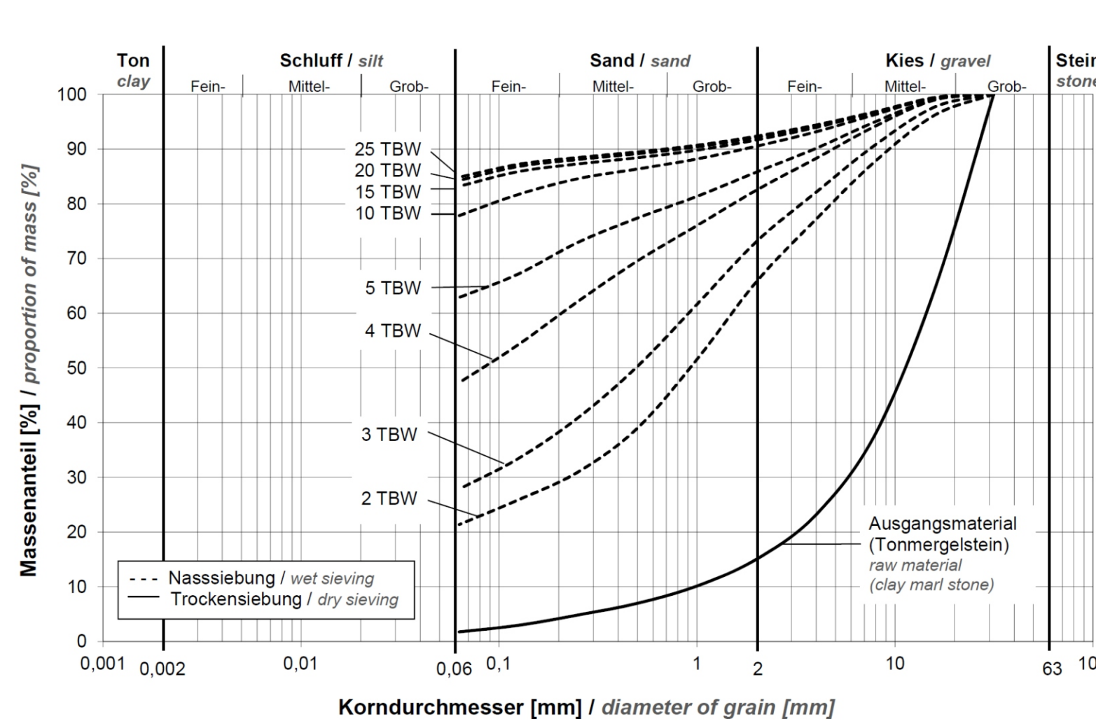
Trocknungs-Befeuchtungs-Wechsel (TBW) kombiniert mit Siebanalysen bei ausgewählten Zyklen zur quantitativen Bewertung Drying-wetting cycles combined with sieve tests at selected cycles for quantitative assessment
