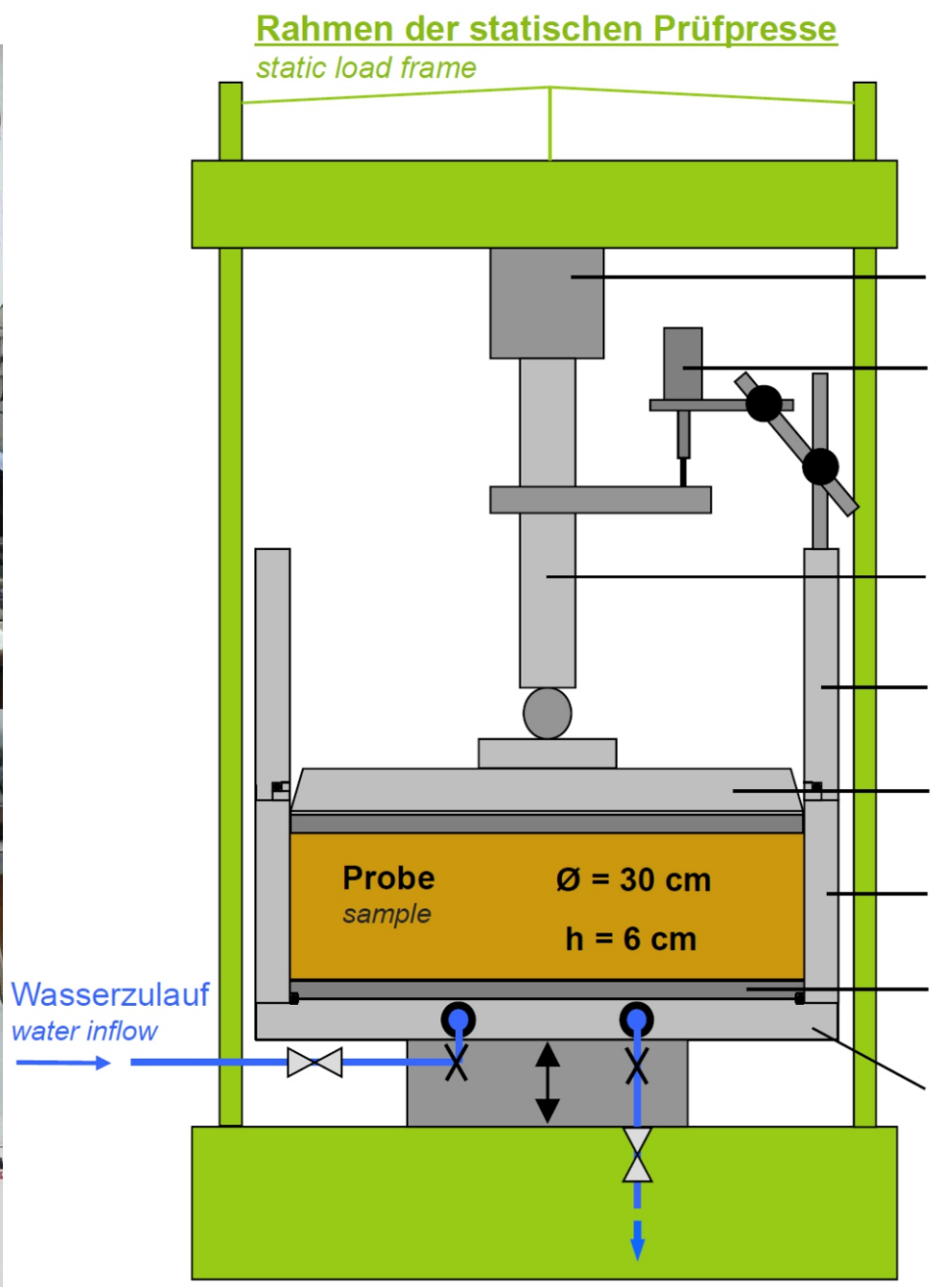
Eindimensionaler Kompressionsversuch - Versuchsgerät und schematischer Versuchsaufbau One dimensional oedometer test - cylindrical oedometer and schematic experimental setup
