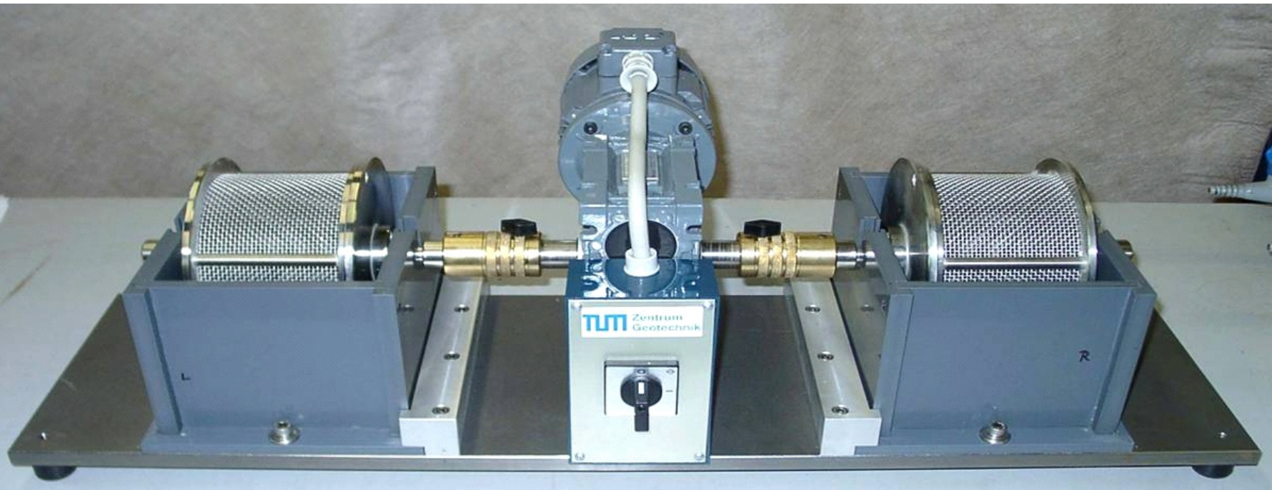
Siebtrommelversuch - Versuchsgerät Slake Durability Equipment
