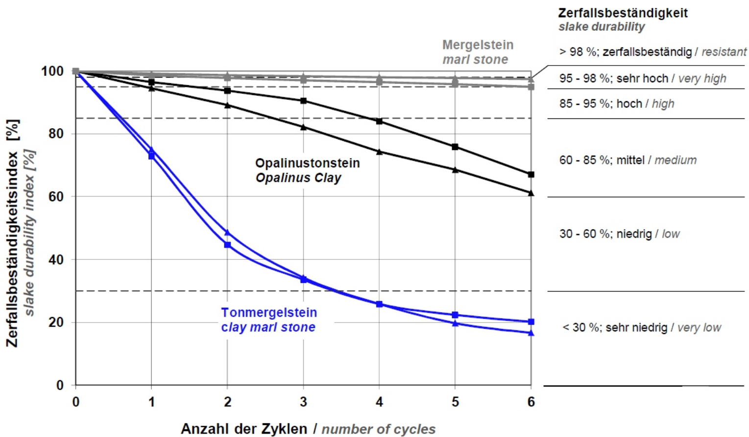
Siebtrommelversuch - Auswertung nach Empfehlung Nr. 20, AK 3.3 "Versuchstechnik Fels", DGGT Slake Durability Test - Evaluation on the Recommendation no. 20, commission on "Rock Testing", DGGT
