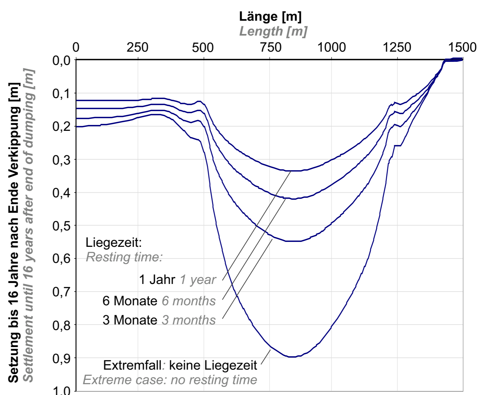
Prognoseergebnisse zeigen den großen Einfluss der Liegezeit auf die darauf folgende zeitabhängige Setzung Results of the simulation show the strong influence of the resting time on the time-dependent settlement
