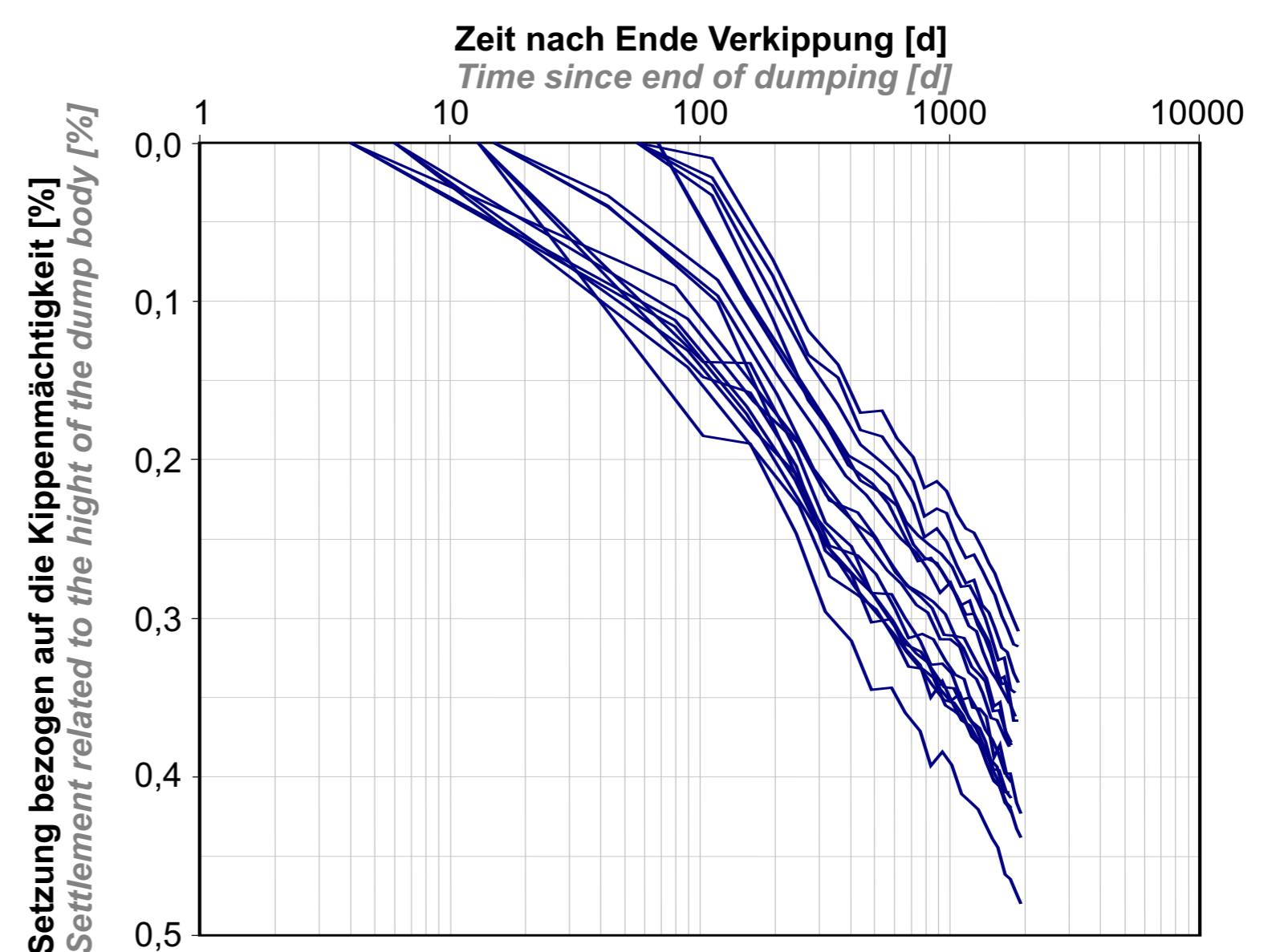
Eigensetzung einer Kippe aus überwiegend locker gelagerten Sanden Settlement under self-weight of dumped and loose coarse grained soils
