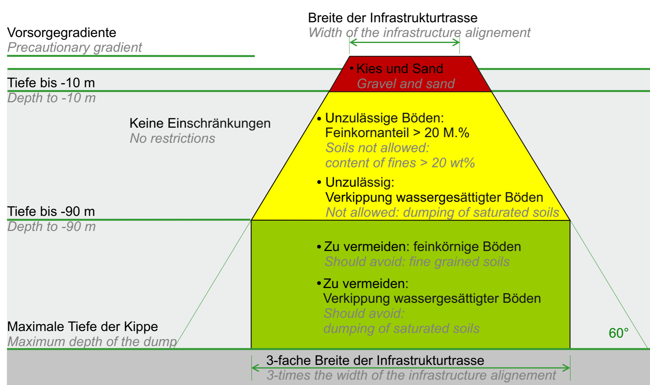
Verkipfungskonzept zur Reduzierung des Setzungspotentials Dumping concept for reducing potential settlements
