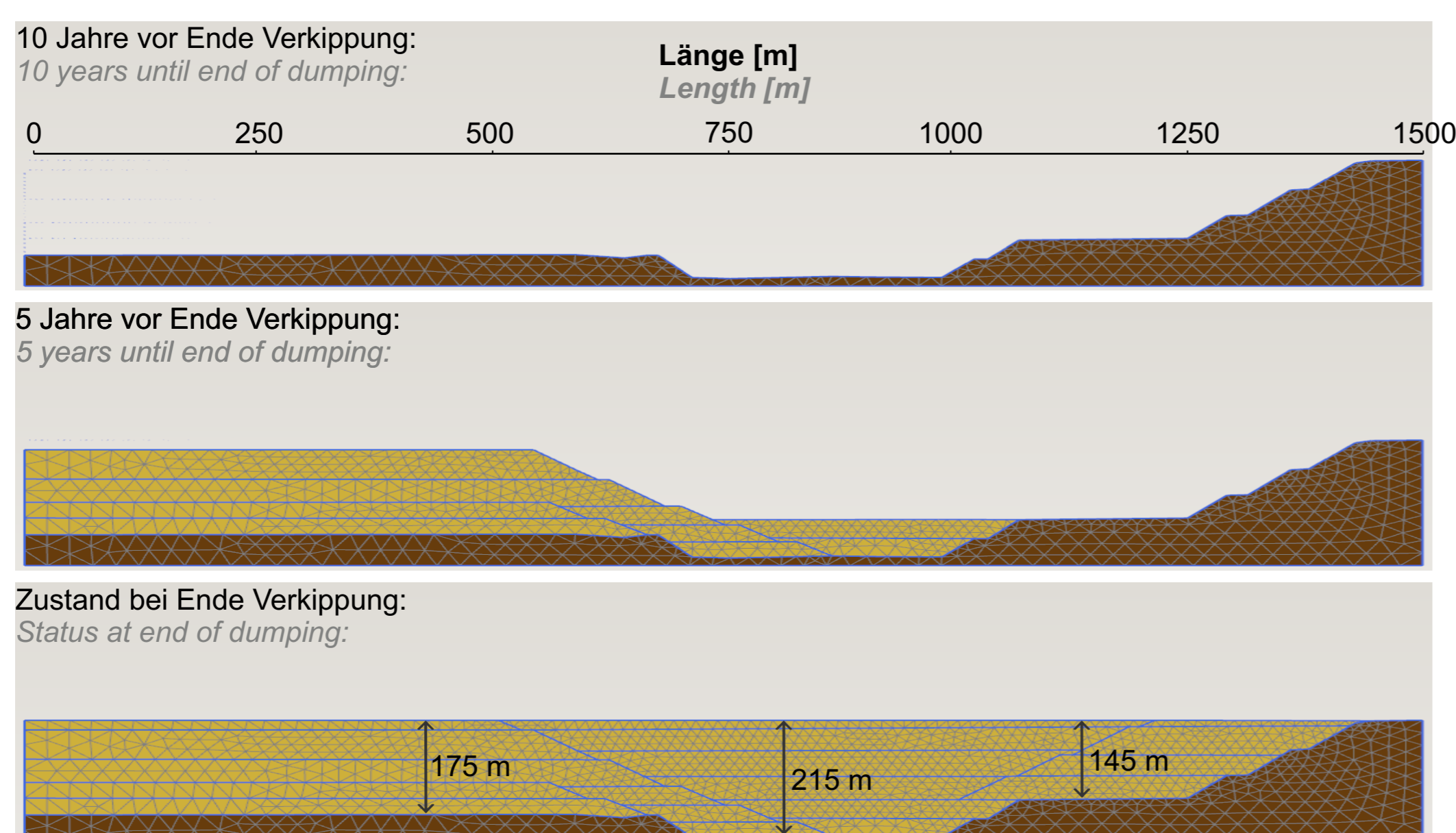
Beispielhafte Simulation eines Verkipfungsprozesses und Prognose der Kippeneigensetzungen mit der Finiten-Elemente Methode und einem visko-plastischen Stoffmodell Exemplary simulation of a dumping process and prediction of settlements under self-weight by using the Finite-Element method and a visco-plastic soil model
