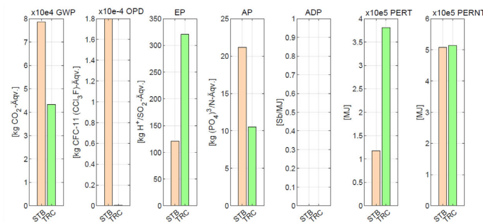
Abb. 5: Vergleich einer konventionellen Verstärkung mit einer Stahlbetonschicht (STB) und einer Verstärkung mit Carbonbeton (TRC) hinsichtlich des globalen Treibhauspotentials (GWP), des Abbaupotentials der Ozonschicht (OPD), des Eutrophierungspotentials (EP), der Versauerung (AP), des erneuerbaren Primärenergiebedarfs (PERT) und des nicht-erneuerbaren Energiebedarfs (PERNT), aus [9]
