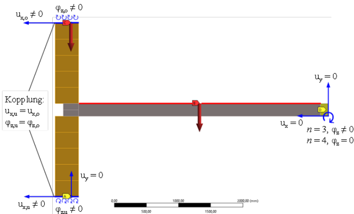
Abb. 8: Rahmenerersatzsystem der Parameterstudie als vereinfachtes 2D-Mikromodell mit Angabe der Lagerungsbedingungen und Freiheitsgrade
