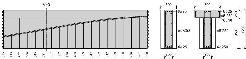
Abb. 5: Konstruktive Durchbildung der vorgespannten Balkenelemente, Spann- ligengeometrie, Rechteckquerschnitt, Plattenbalkenquerschnitt
