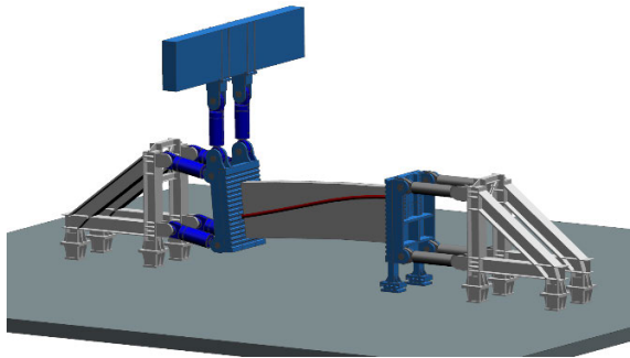
Abb. 1: Versuchskonzept mit Balkenelement und angedeuteter Spanngliedführung
