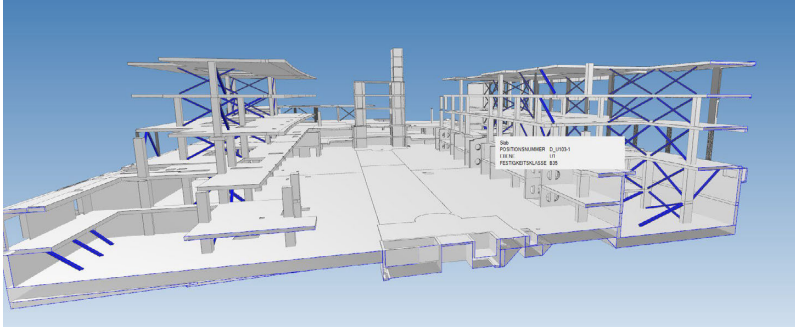
Abb. 5: Visualisierung Abbruchzustand inkl. Hilfsaussteifung (BIM Modell Tragwerk)
