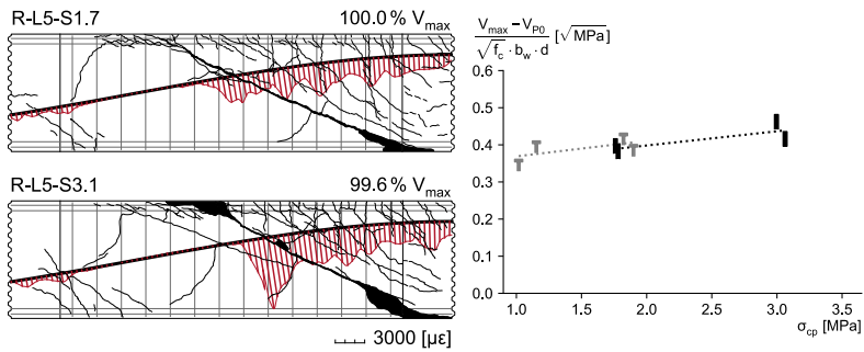
a) Bruchbild zweier Balkenelemente mit Dehnungsprofil des Spannglieds
