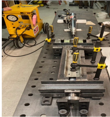
Abb. 2: Vorspannen der mit Glasfaser versehenen Litzen in einer Rahmenkonstruktion im DYWIDAG Prüflabor Leipzig
