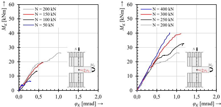
Abb. 7: Experimentelle Moment-Rotations-Diagramme in Abhängigkeit der Wandnormalkraft N und einer Aufteilung des Einspannmoments M_K von jeweils 50 % in Wandfuß- und Wandkopfquerschnitt
