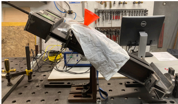
Abb. 3: Verpressen der mit Glasfaser versehenen Einzellitzenspannglieder im DYWIDAG Prüflabor Leipzig
