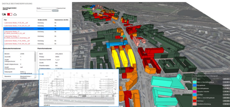
Abb. 4: Bestandsmodell – Ausschnitt Haltestellen Borgweg bis Jarrestraße: Formular- und modellbasierte Abfrage von Informationen (Visual Reporting)
