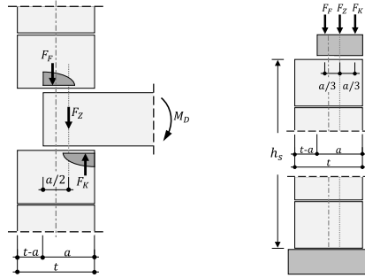
Abb. 3: Belastungssituationen am Außenwand-Decken-Knoten infolge teilauf- liegender Decke und daraus abgeleitete Teilflächenbelastungen
