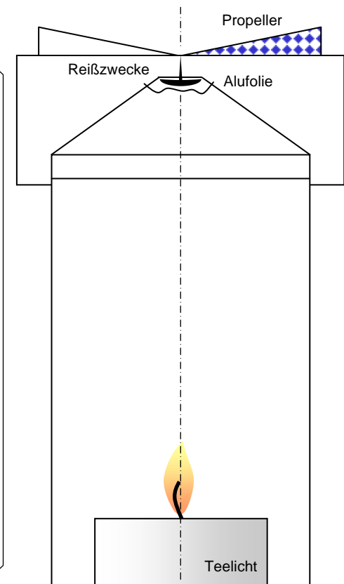
Querschnitt
